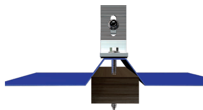
Схема установки кронштейна MR-VI-01 на мягкую кровлю
