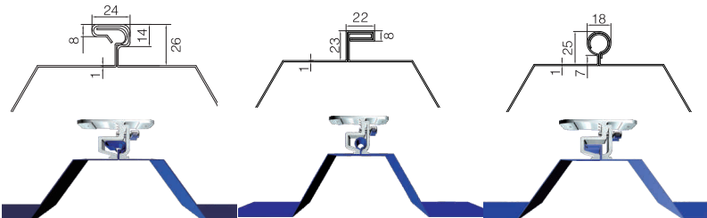
Схема установки кронштейна XMR-VI-11
