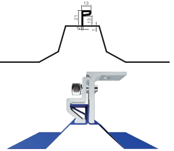
Схема установки кронштейна XMR-VI-08
